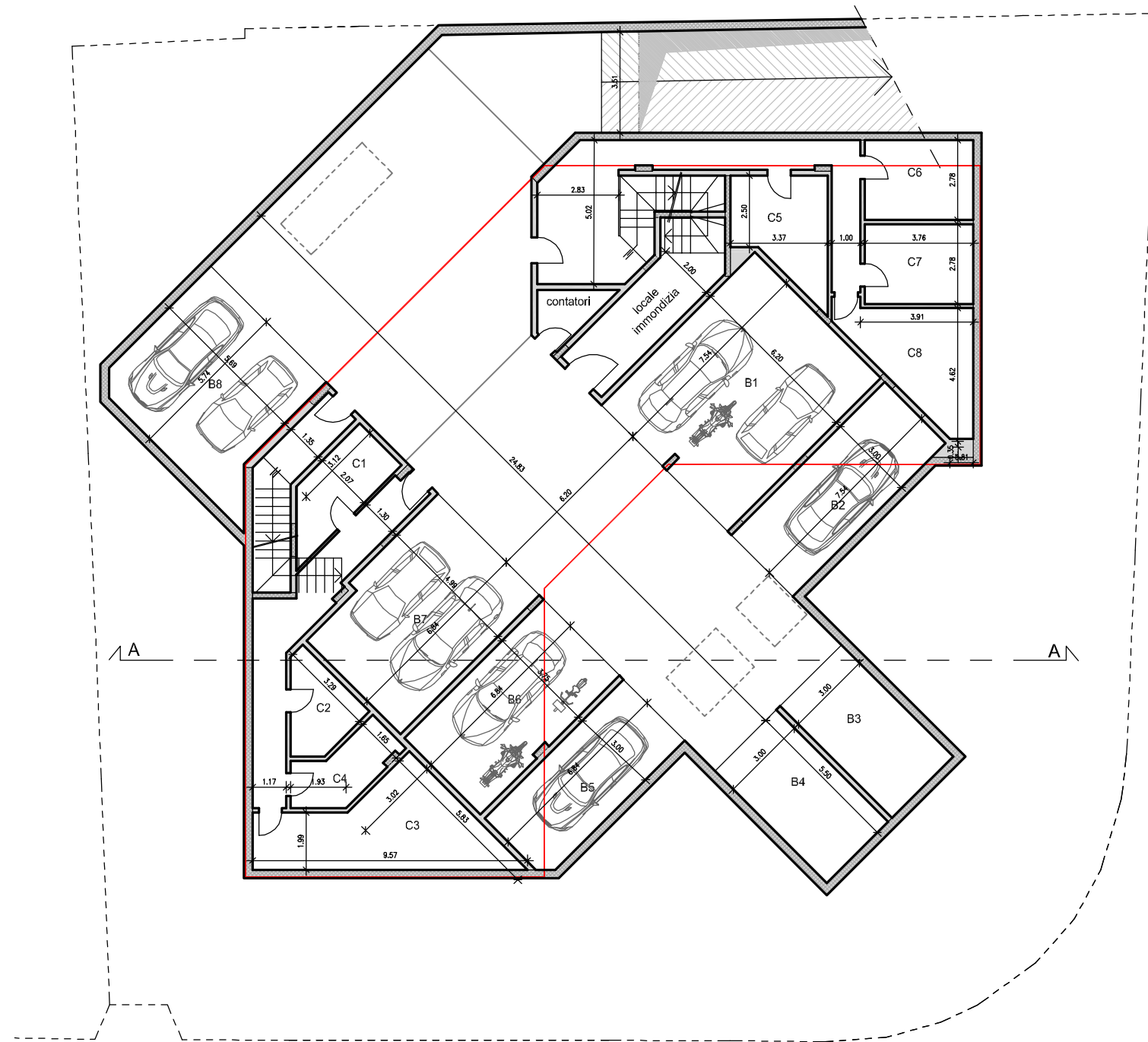
PIANO INTERRATO scala 1:200
